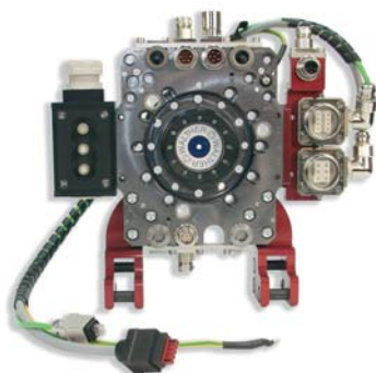
Type 91489-0 Werkzeugseite / tool-side
