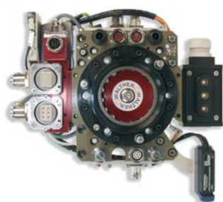
Type 91489-2 Roboterseite / robot side
