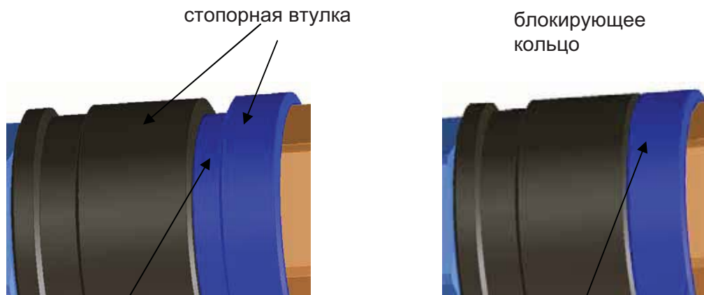
рисунок 1 заблокированное положение
