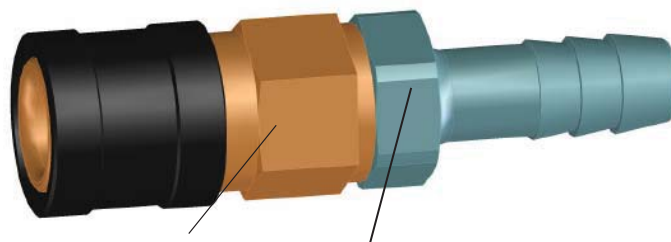
корпус БРС шестиугольного сечения шестиугольный соединительный элемент (предоставлен заказчиком)
